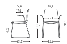
Cantilever with simple arm Patín metálico con brazo simple
