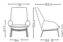
4 Metal legs chair 4 Patas metálicas
