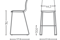
Cantilever stool without arms Taburete patín metálico sin brazos
