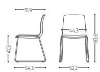
Cantilever without arms Patín metálico sin brazos
